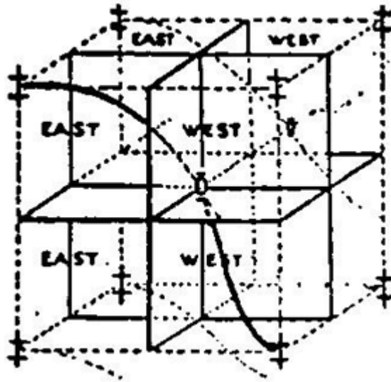
Fig. 48 Les six miroirs intérieurs de la radiation.
