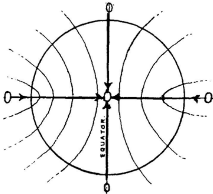
Fig.61. Illustrant la nature bilatérale de la matière et l'apparente courbure de la gravité.
