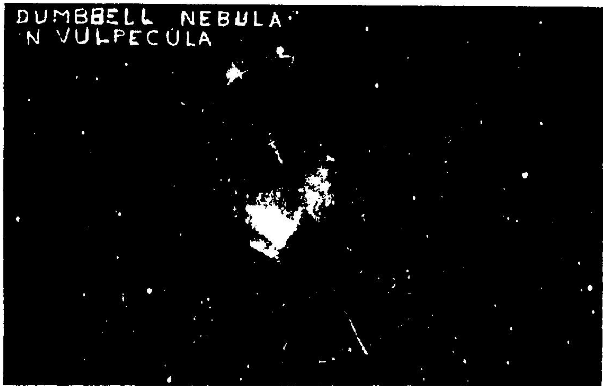
Fig. 148. Illustrant le principe de la mort dans toutes les matières. Les sphères sont créées en comprimant des anneaux pour les former. Les sphères sont ensuite désintégrées en projetant des anneaux jusqu'à ce qu'un trou noir entoure leur axe de rotation et elles s'agrandissent progressivement jusqu'à disparaître dans leurs cathodes.
