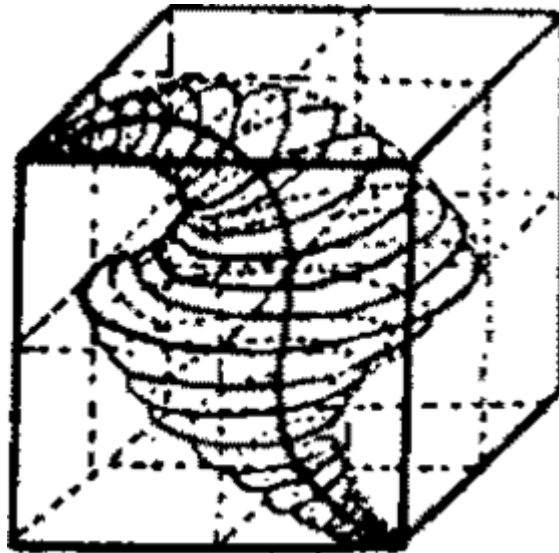
Fig. 49. Spirales d'ondes sur leur axe d'onde
