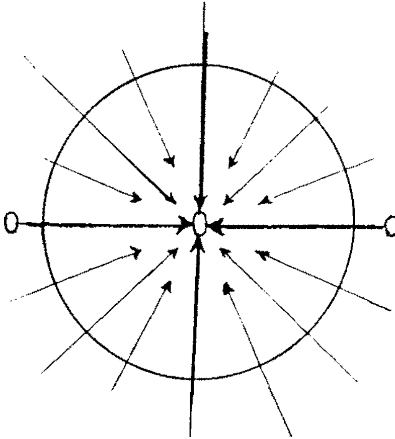
Fig. 59 Illustrant le concept d'univers radial.
